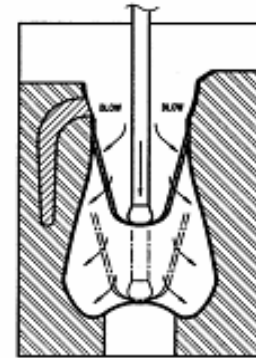
(프리폼을 연신봉으로 연신하여 성형하는 공정)
