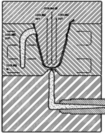
(프리폼을 성형하기 위해 수지를 주입하는 공정)
