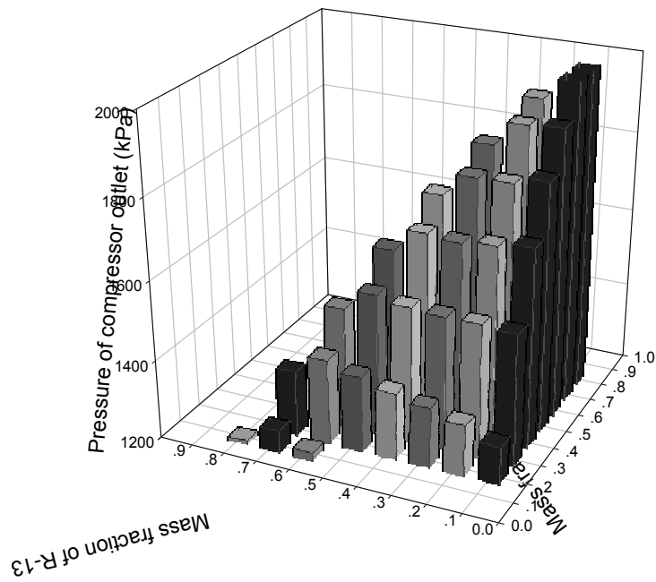
(d) Pressure of compressor outlet
